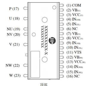
PIN1-PIN23
