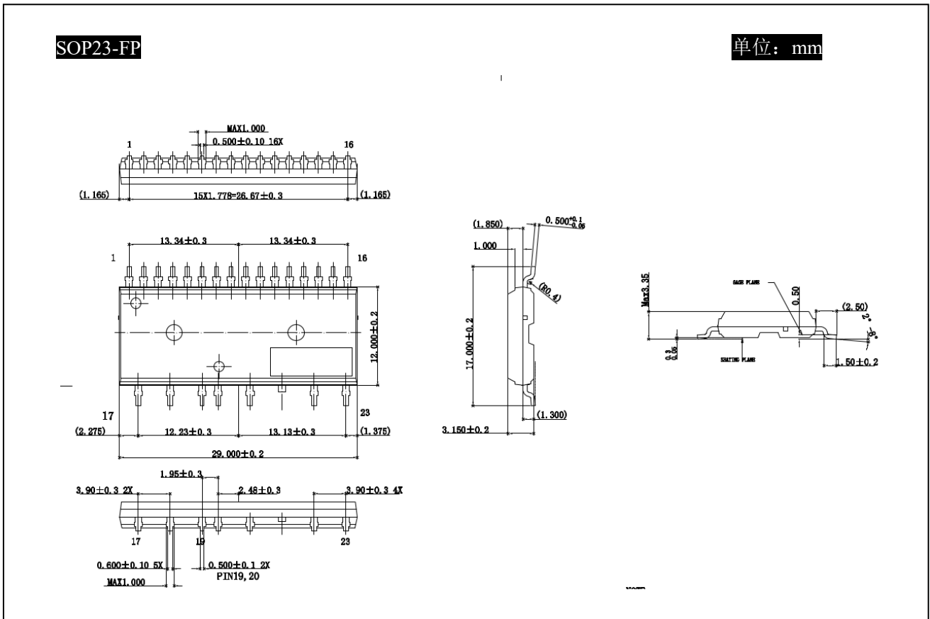
图 11: 封装外形图
